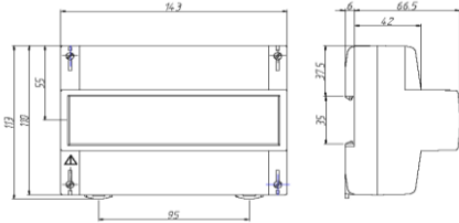
Рисунок 1 - Загальний вигляд лічильника ЦЭ6804-U у корпусі P31
