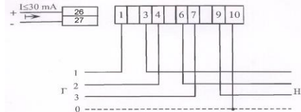
Рисунок 2 - Схема підключення лічильника ЦЭ6804-U у корпусі P31
