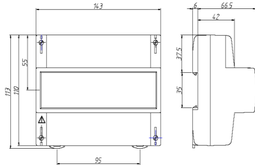
Рисунок 1 - Загальний вигляд лічильника ЦЭ6804-U у корпусі РЗ1
