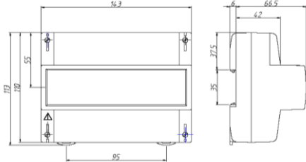
Рисунок 1 - Загальний вигляд лічильника ЦЭ6804-U у корпусі РЗ1
