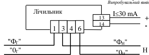
Рисунок 2 – Схема підключення лічильника ЦЭ6807Б-У в корпусі ШБ
