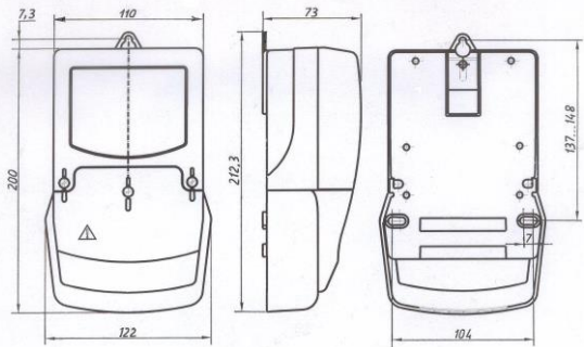
Рисунок 1 - Загальний вигляд лічильника CE102-U в корпусі S7
