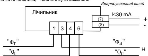
Рисунок 3 - Схема підключення лічильника CE102-U в корпусі S7
