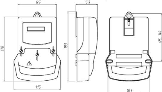
Рисунок 1 - Загальний вигляд лічильника CE102-U в корпусі S6
