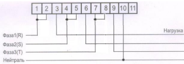
Рисунок 2 - Схема підключення лічильника CE303-U в корпусі R33
