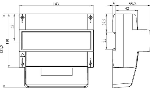
Рисунок 1 - Загальний вигляд лічильника CE303-U в корпусі R33
